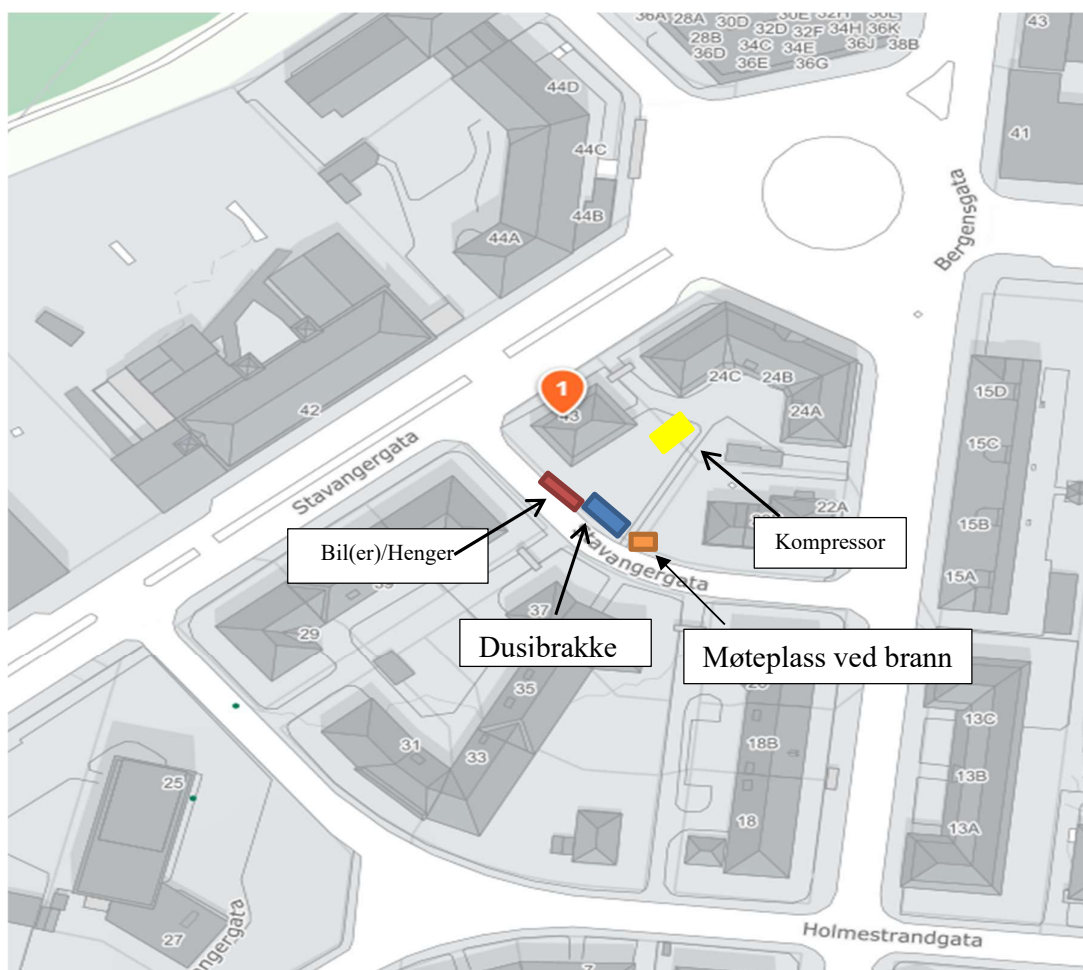
OVERSIKTSKART BYGGEPLASS (RIGGPLAN)
